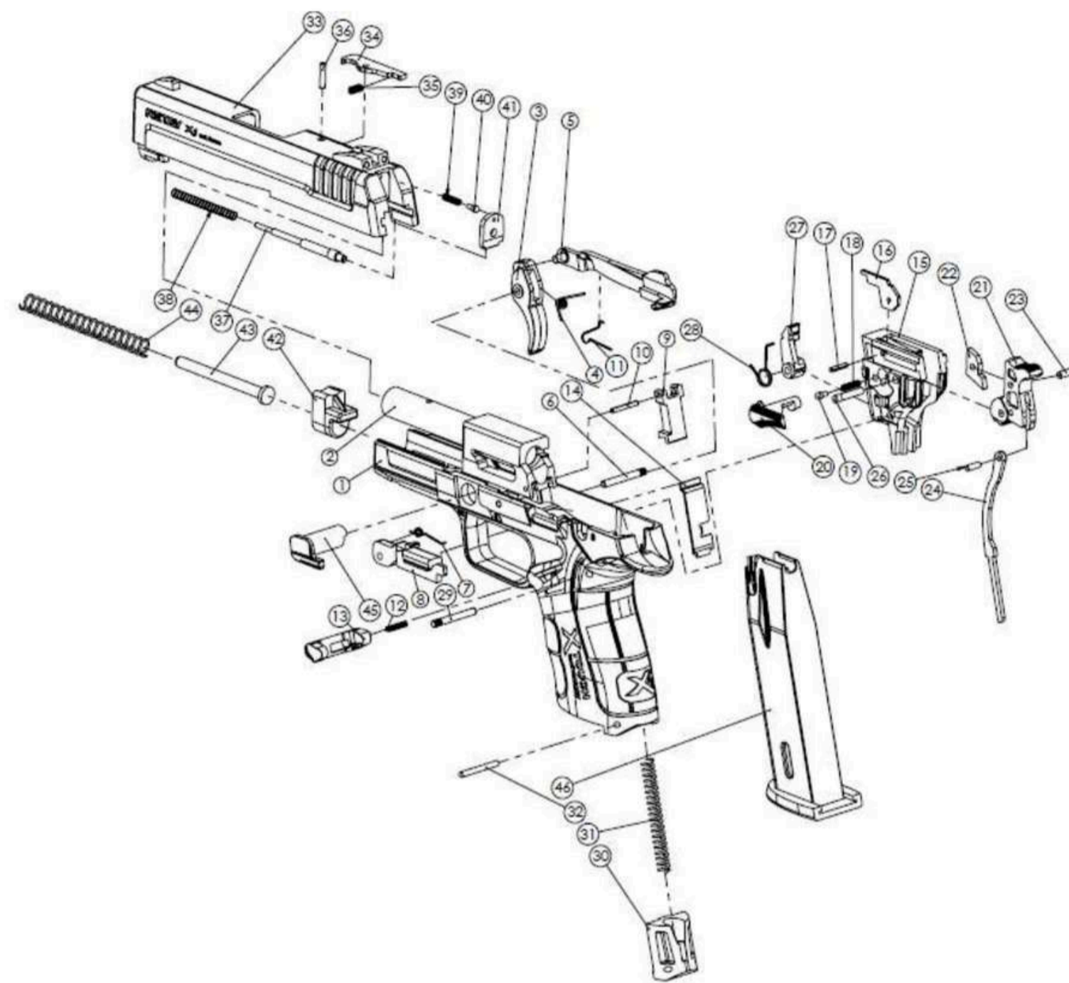
Pistol 9mm
